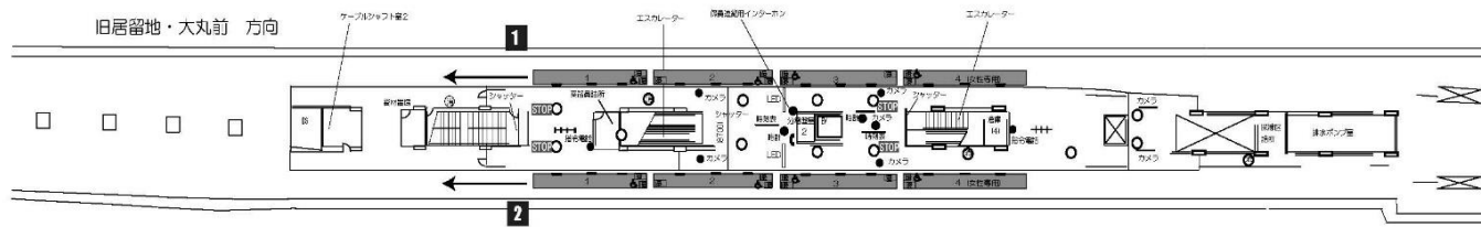
地下3階平面図
