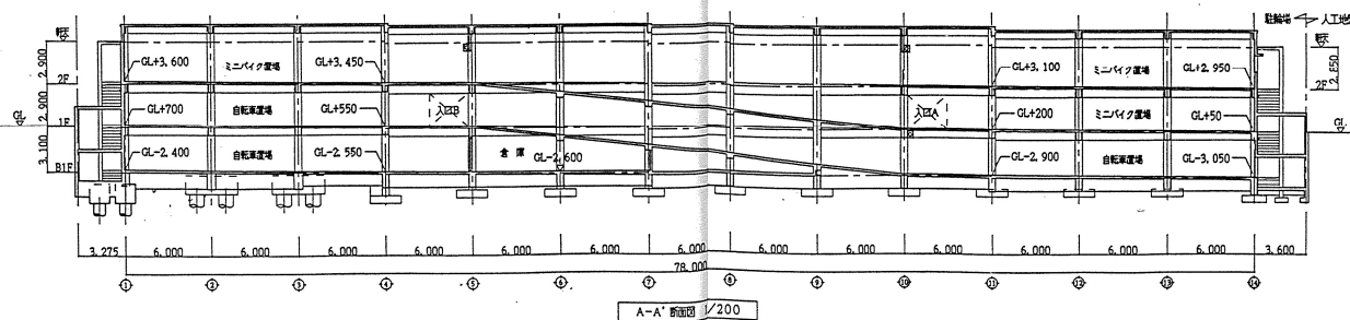
A-A'断面図 1/200
