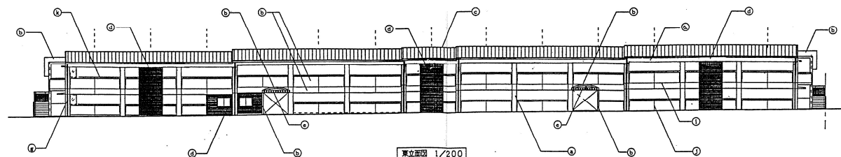
東立面図 1/200
