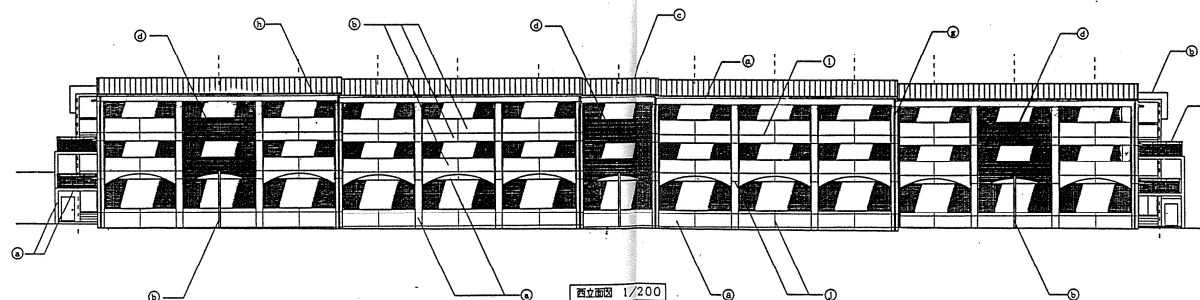
西立面図 1/200
